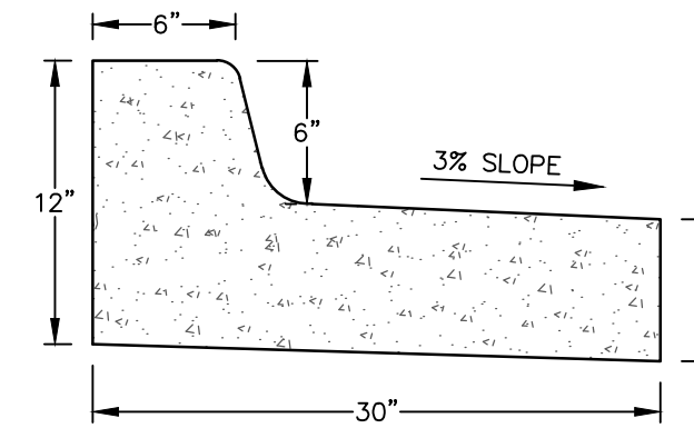
SPILL TYPE CURB & GUTTER N.T.S.
