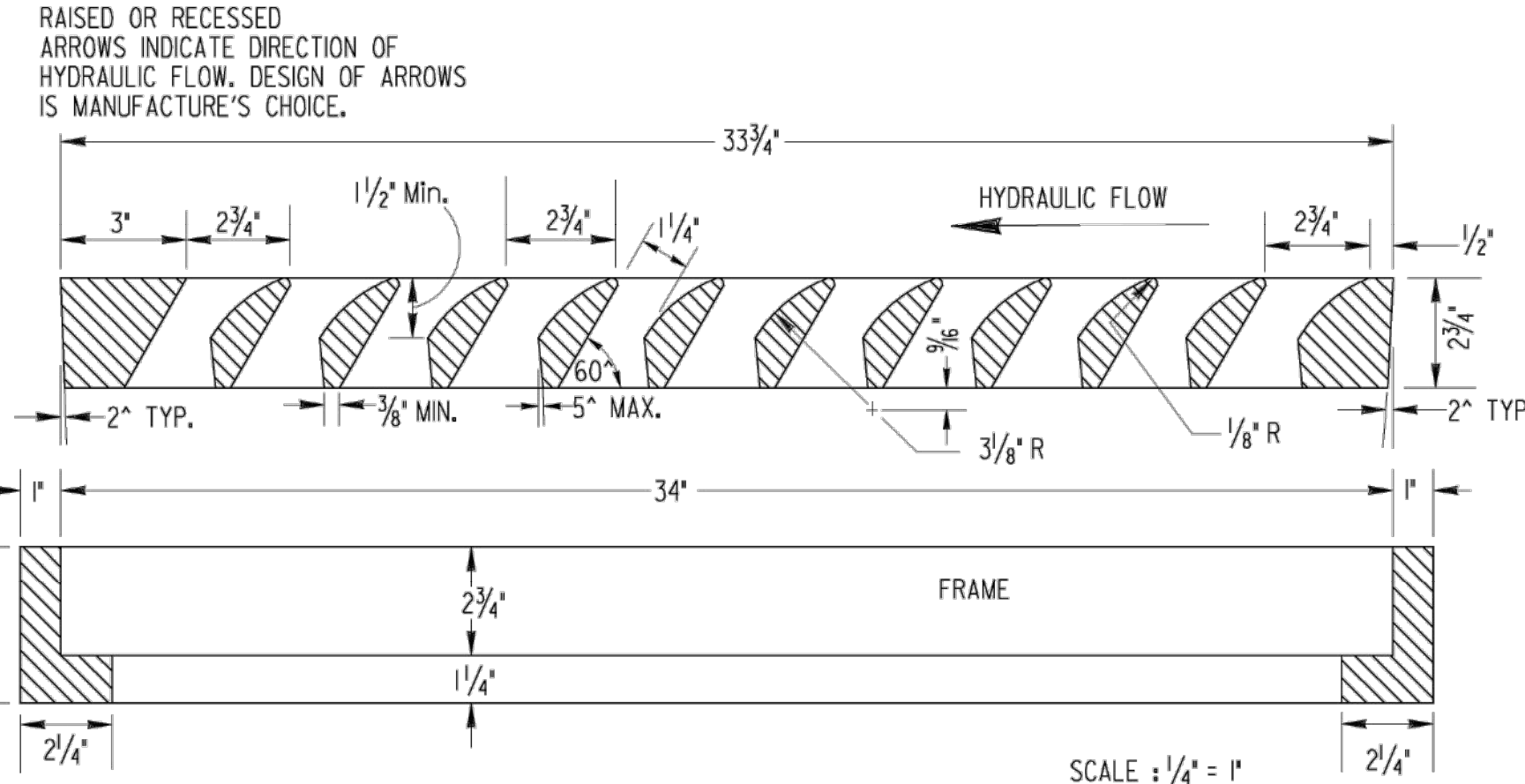
SECTION C-C SCALE: 1/4" = 1"
