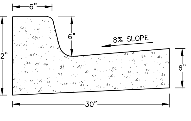
STANDARD TYPE CURB & GUTTER N.T.S.
