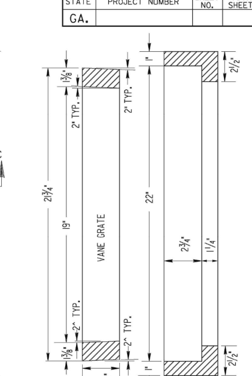
SECTION D-D
