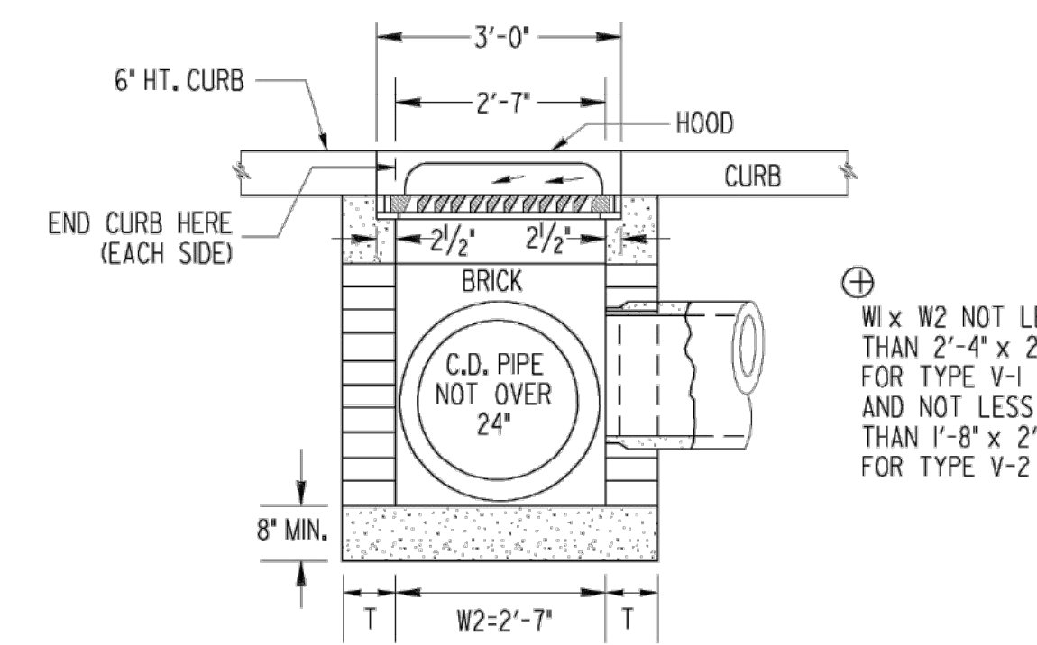
SECTION B-B SCALE: 1/2" = 1 FT.
