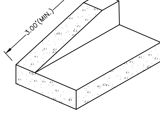
CURB TERMINATION DETAIL N.T.S.
